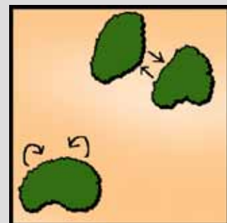
ככל שהמרחק בין הכתמים קטן יותר, רב הסיכוי שיתקיימו קשרי גומלין בין פרטים ומינים החיים בכתמים סמוכים
