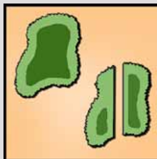
ערכו של כתם שלם לשימור מגוון ביולוגי גדול יותר מערכו של כתם מקוטע בגודל דומה
