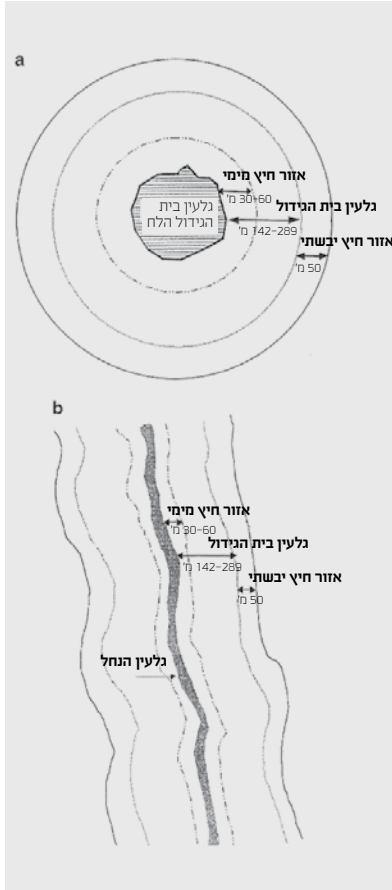
הצעה לתכנון אזורי חיץ לשימור (a) מקווי מים; (b) נחלים (Semlitsch & Bodie, 2003). שני סוגים של אזורי חיץ מוכלים בתחום שבין קו המים ועד למרחק 289 מטרים ממנו: אזור חיץ מימי שמטרתו לשמור על איכות המים, ואזור גלעין בית הגידול שאמור לספק בתי גידול לשלבים שונים במחזור החיים של דו-חיים חצי-יבשתיים וזוחלים מימיים. אזור החיץ היבשתי מספק מעטפת נוספת של הגנה על אזור הגלעין השמור מפני השפעות שוליים.
