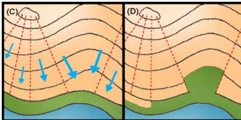
תכנון רחובו של אזור החיץ על-פי התנאים הטופוגרפיים ועוצמת הזרימה של הנגר העילי. האיור השמאלי מציג את ההבדלים בעוצמת הנגר העילי בנקודות שונות לאורך שולי הערוץ, והאיור הימני מציג עקרונות להתאמת מקומית של רוחב החיץ המשמר לתנאים הטופוגרפיים (מתוך Bentrup, 2008).
