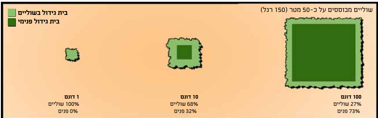
ככל שהכתם הטבעי גדול יותר, הוא יכול אחז גבוה יותר של "בתי גידול פנימיים" שאינם מושפעים מאפקט השוליים. בתי הגידול הפנימיים חשובים לשימור מינים הרגישים להפרעות ולקיטוע של בתי גידול טבעיים. (מתוך Bentrup 2008)
